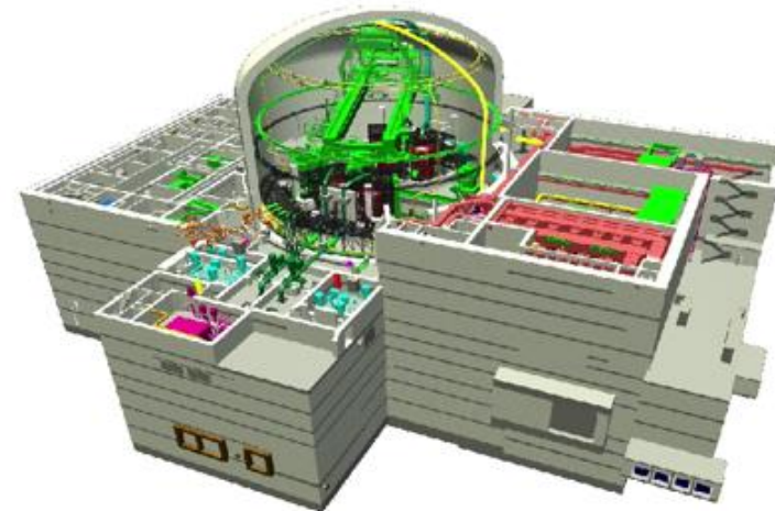
(1) Source : Vue 3D Bâtiment réacteur EPR 2 Edvance - ElectricDays
